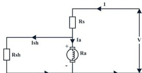
Gambar 6. Rangkaian Ekuivalen Motor Kompon Pendek
