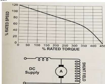
Gambar 4. Karakteristik Motor Kompon DC
